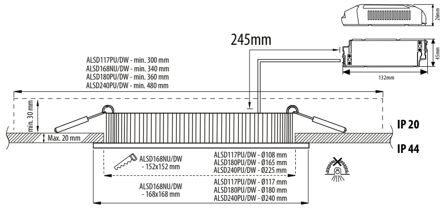
Velox-paneelien mitoitus upposennuksessa
